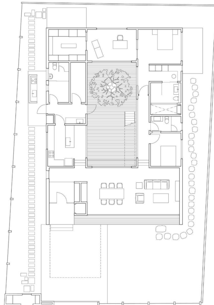
План жилого дома с внутренним двориком
