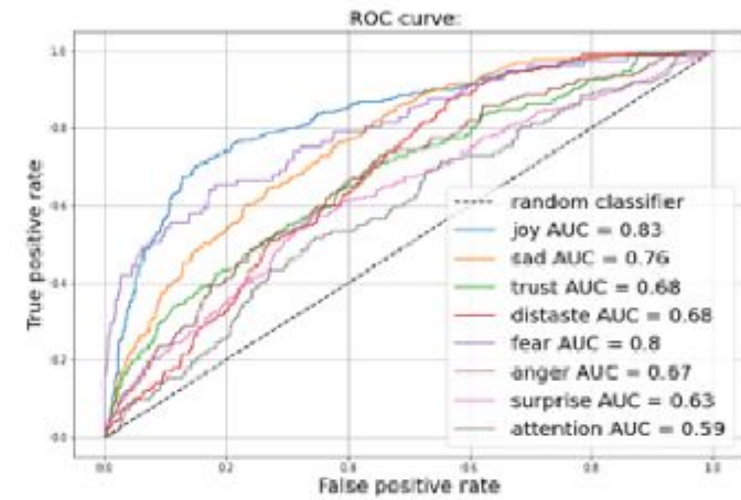
Анализ тональности текстов
